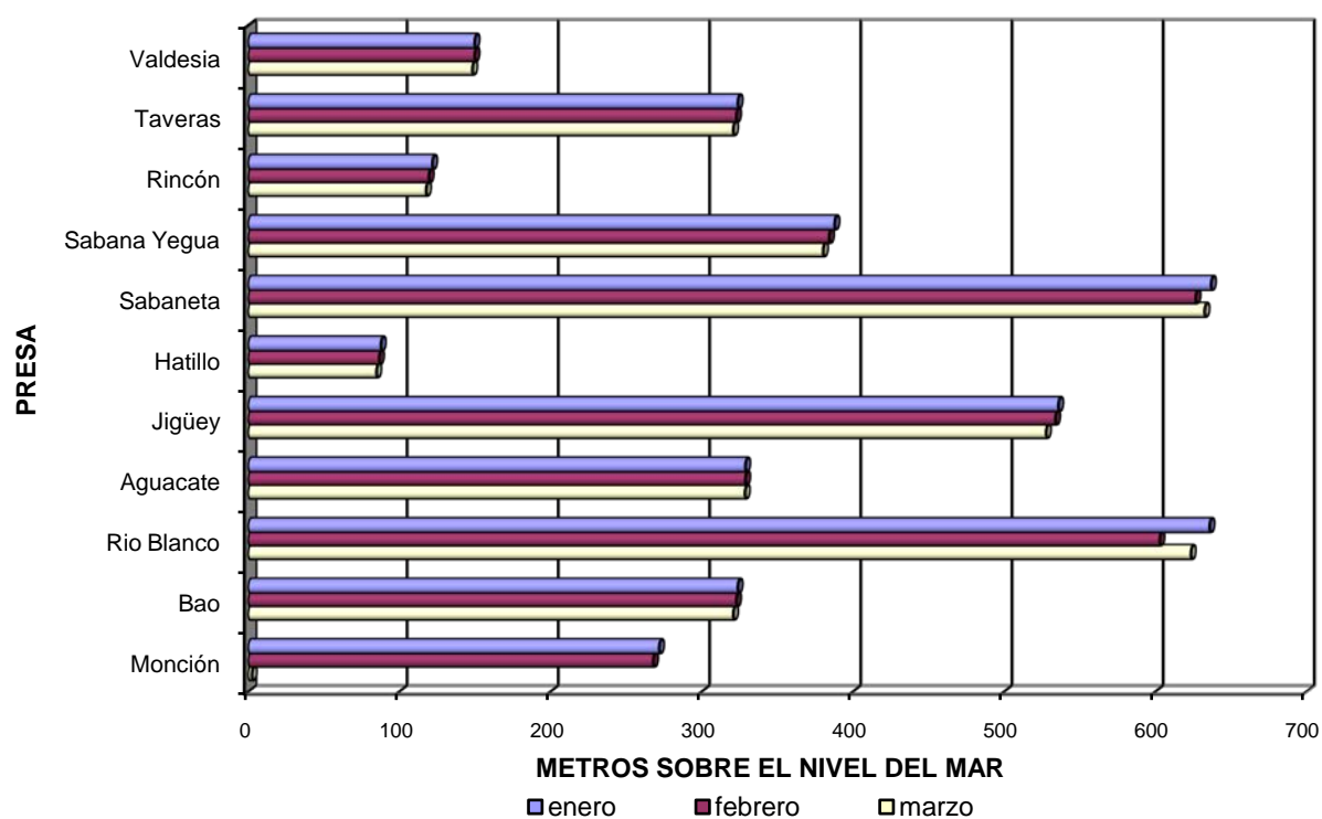
Promedios Mensuales del Nivel de Agua en los Embalses del País: enero-marzo 2007
