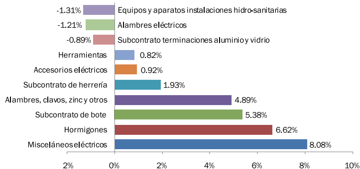
Gráfico 6 REGIÓN METROPOLITANA: Variación porcentual mensual del Índice de Costos Directos de la Construcción de Viviendas, según subgrupos de costos, en el mes de agosto del 2018
