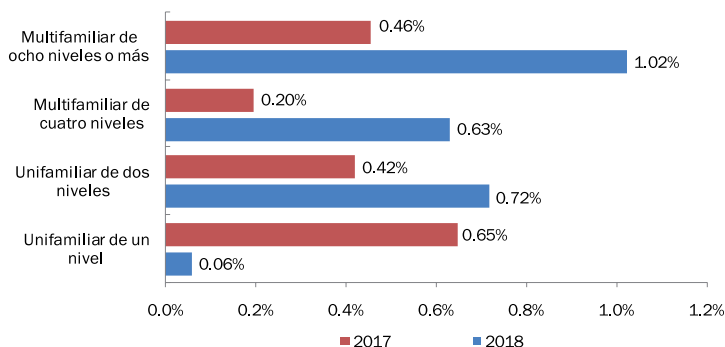
Gráfico 4 REGIÓN METROPOLITANA: Variación porcentual mensual del Índice de Costos Directos de la Construcción de Viviendas, según tipos de viviendas, en el mes de agosto del 2017 y 2018
