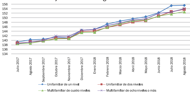
Gráfico 3 REGIÓN METROPOLITANA: Índice de Costos Directos de la Construcción de Viviendas, según tipos de viviendas, de julio del 2017 a agosto del 2018
